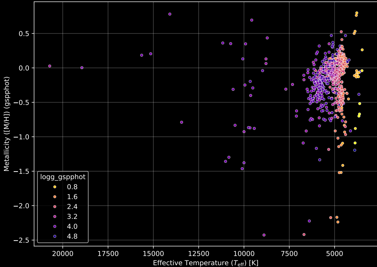
APOGEE DR17 Field: [K19_076+07] Stellar Population Parameters (n= 751)
